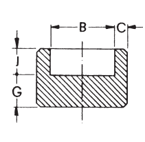
tappi femmina
