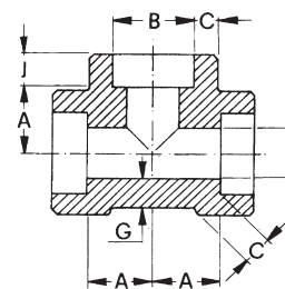
tee
