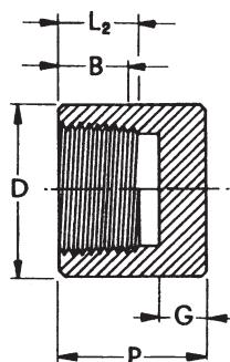
tappi femmina
