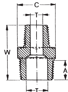
nippli esagonali ridotti To BS 3799
