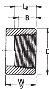
mezzi manicotti
