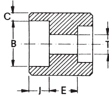
manicotti ridotti
