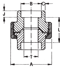
bocchettoni F/F
