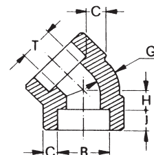
gomiti 45°
